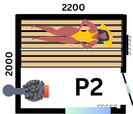
MODELL GERÄUMIG (P2)
